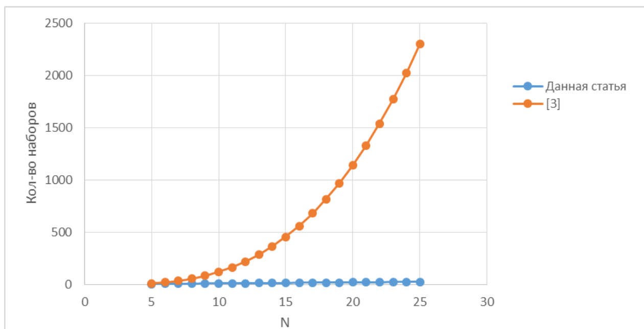
Рисунок 1 - График роста количества наборов при фиксированном t=3
