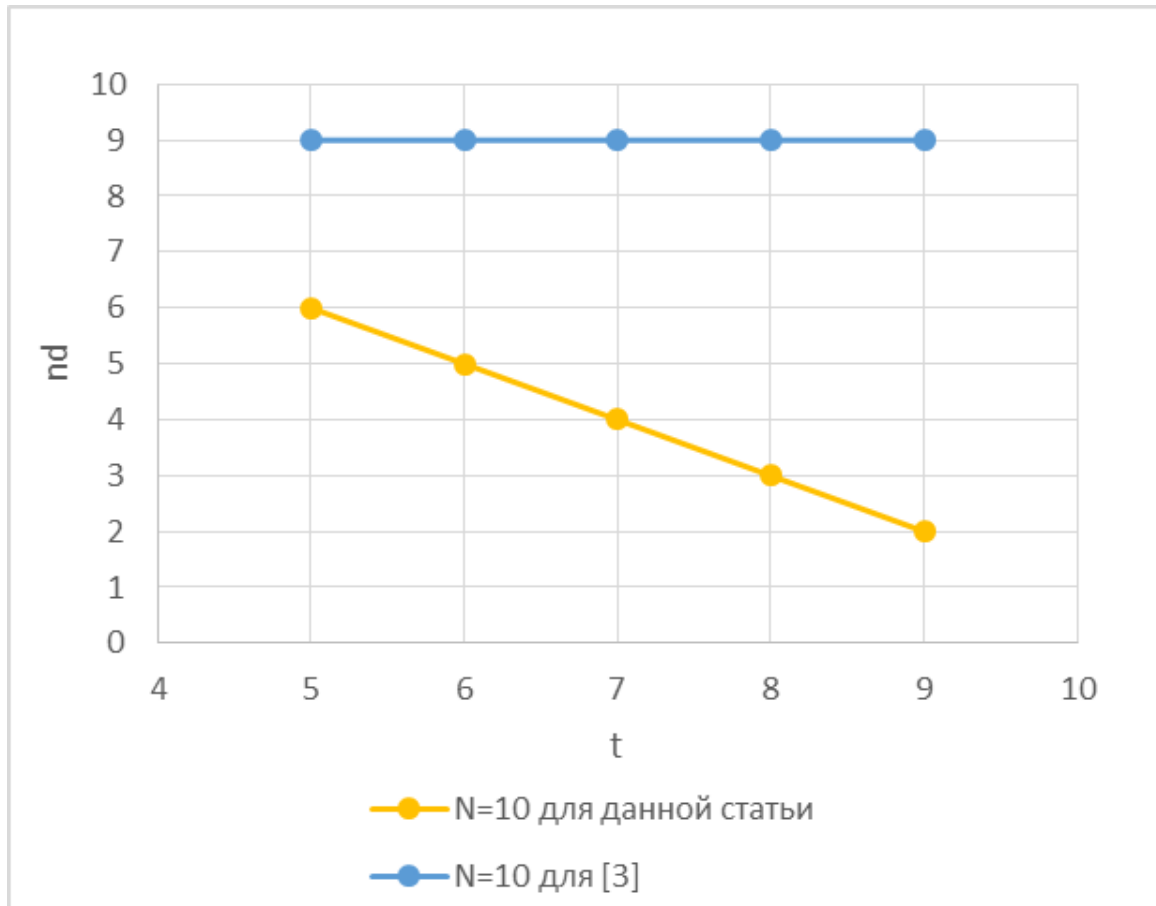
Рисунок 2 – Зависимость количества долей в наборе от порогового числа
